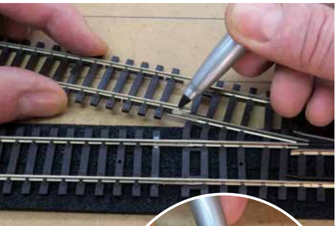
4 Dans ce cas, le rail situé à l'intérieur de la courbe doit être recoupé. On repère le trait de coupe à l'aide d'un marqueur à encre indélébile.
