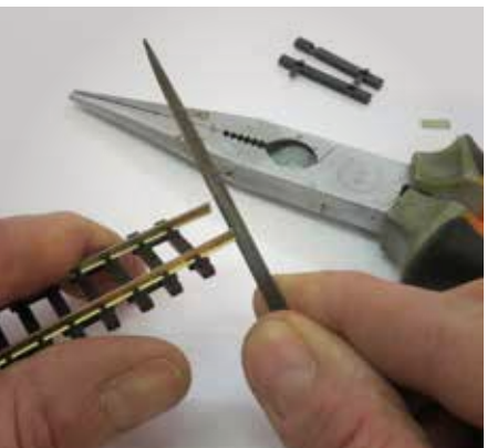
7 Un petit coup de lime est nécessaire pour obtenir une tranche bien nette.
