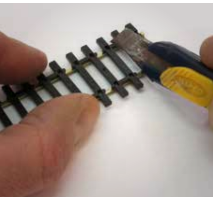
5 Pour sectionner le travelage, un coup de cutter suffit.
