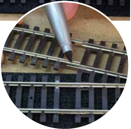
4 Dans ce cas, le rail situé à l'intérieur de la courbe doit être recoupé. On repère le trait de coupe à l'aide d'un marqueur à encre indélébile.
