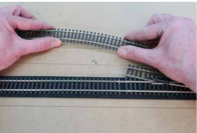
3 Sur cet exemple, il s'agit de créer une contre-courbe en utilisant une voie courbable.
