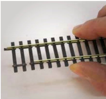
2 Si l'on cintré une voie courbable, le rail situé à l'extérieur de la courbe entre dans le travelage.
