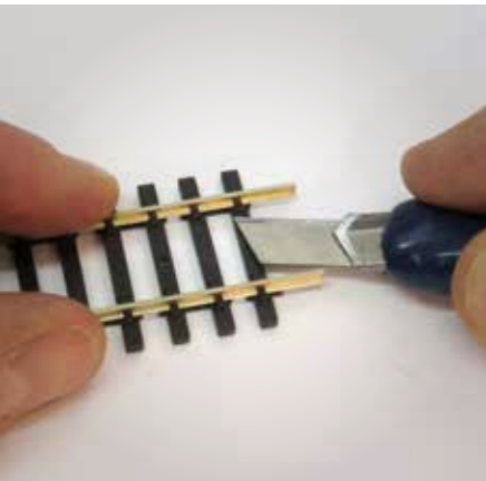
8 Pour glisser les éclisses, il faut supprimer les attaches de rails.
